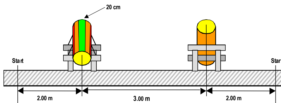
Rys. 22: Ustawienie kozłów do przerzynki kombinowanej
