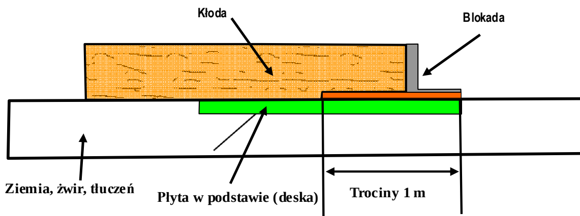
Rys. 33: Deska w podstawie i blokada
