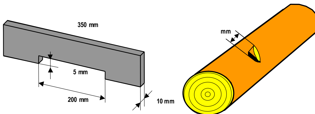
Rys. 39: Wymiary przyrządów pomiarowych i punkty pomiaru
