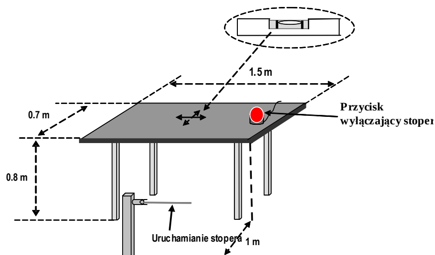
Rys. 20: Stół do konkurencji wymiany piły łańcuchowej
