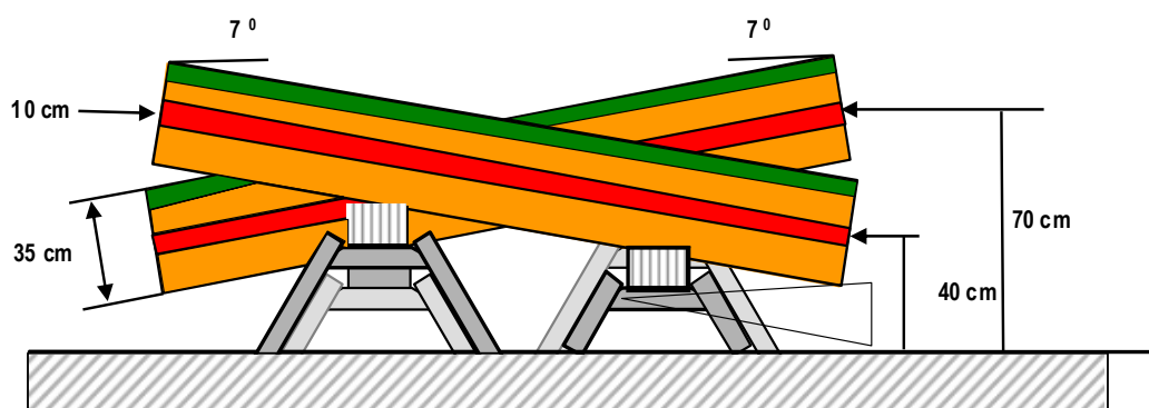
Rys. 21: Ustawienie kłód (kąty) i średnice
