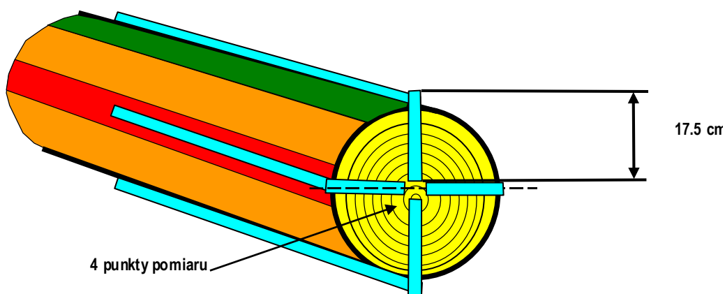
Rys. 23: Pomiary kąta i długość testera
