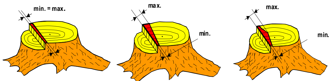
Rys. 14: Szerokość zawiasy
