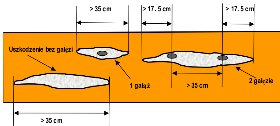
Rys. 43: Uszkodzenia drewna podczas okrzyszowania
