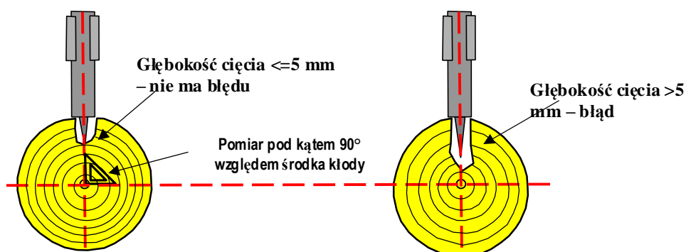
Rys. 41: Pomiar zbyt głębokich cięć, pod kątem 90° względem środka kłody
