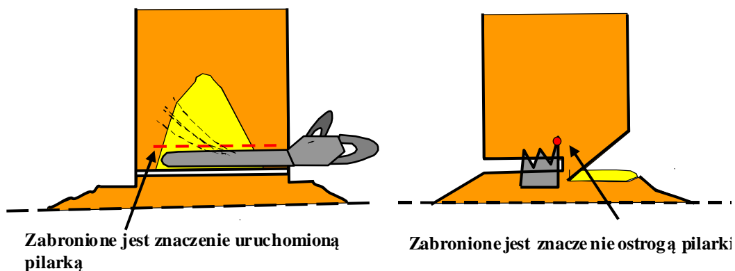
Rys. 5: Zabronione znaczniki
