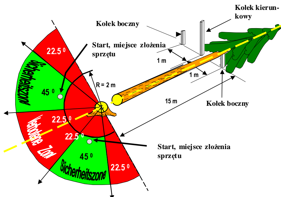
Rys. 6: Kierunek obalania
