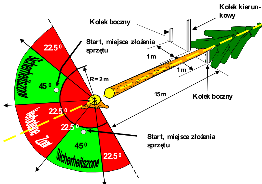
Rys. 6: Kierunek obalania
