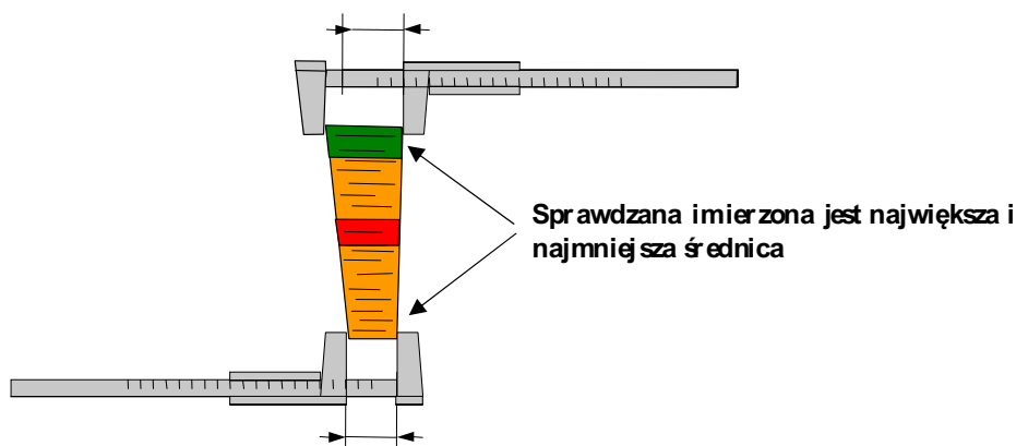
Rys. 30: Mierzenie grubości krążka
