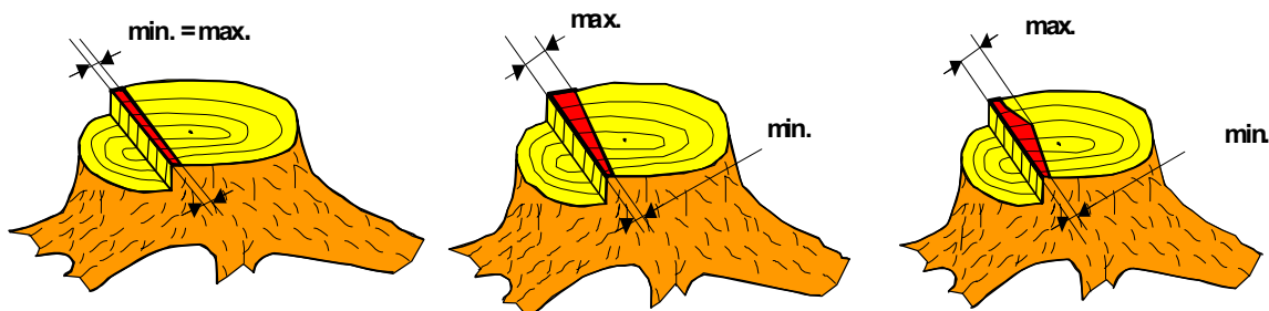
Rys. 14: Szerokość zawiasy
